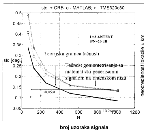
Sl. 5 – Uporedni prikaz teorijske Cramer-Raove granice za grešku procene i greške procene pri implementaciji metode MUSIC u MATLAB-u i signal-procesoru TMS320c30
