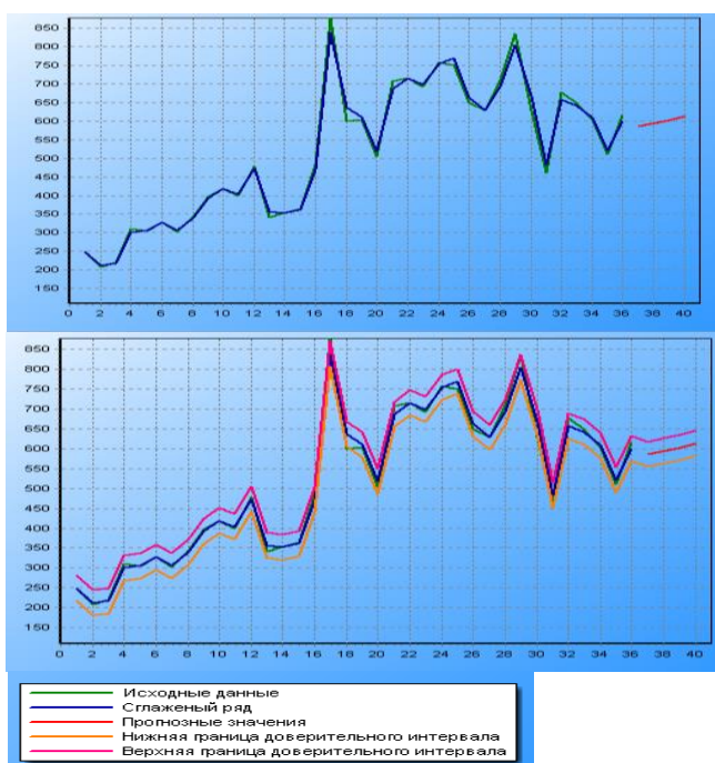
Рисунок 2. Прогнозирование экономического индикатора «кредиты юридических лиц» (представление в виде временных рядов)
