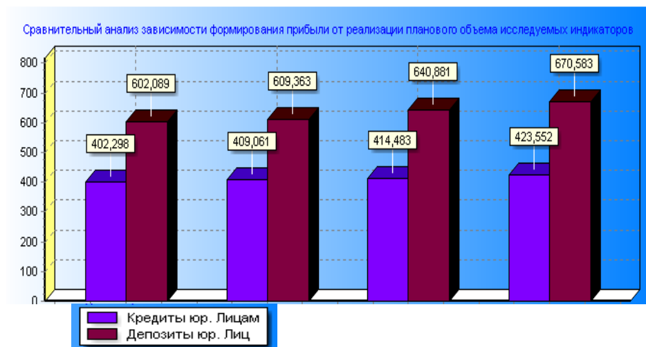
Рисунок 3. Моделируемое значение величины прибыли
