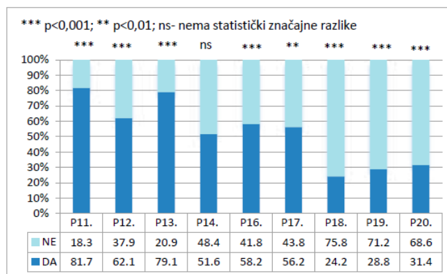
Grafikon 1.
