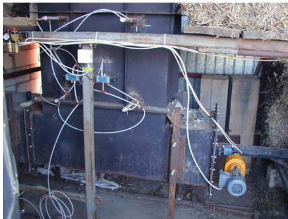
Sl. 2. Spremište (šaržer) bala biomase sa potisnim klipom Fig. 2. Biomass bale repository with the push piston
