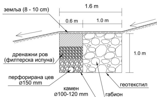
Слика 8 Стабилизационо-дренажна конструкција (излив; ски-стаза „Коњарник 1“, Октобар 2008)
