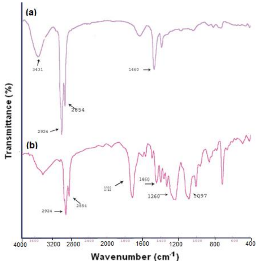
Figure 6. FTIR spectra of (a) virgin and (b) modified asphalt binder Slika 6. FTIR spektri (a) čisto vezivo (b) modifikovano asfaltno vezivo
