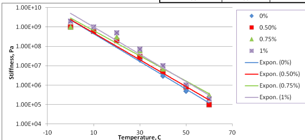
Figure 5. Stiffness modulus at different temperature Slika 5. Modul čvrstoće na različitim temperaturama
