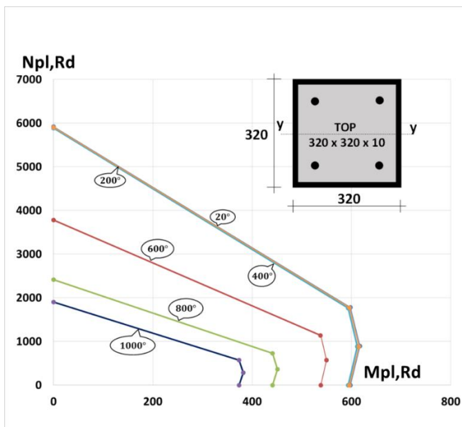
Слика 3: Интеракционе криве за различите температуре шупљег челичног профила испуњеног бетоном
