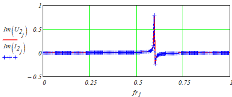
Слика 8 – Имагинарни део – амплитуда померања другог таласног облика Figure 8 – Imaginary part – displacement amplitude of the second waveform
