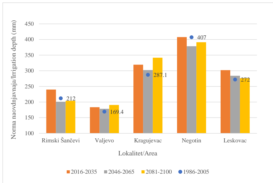
Grafik 3. Norme navodnjavanja kukuruza (mm)
