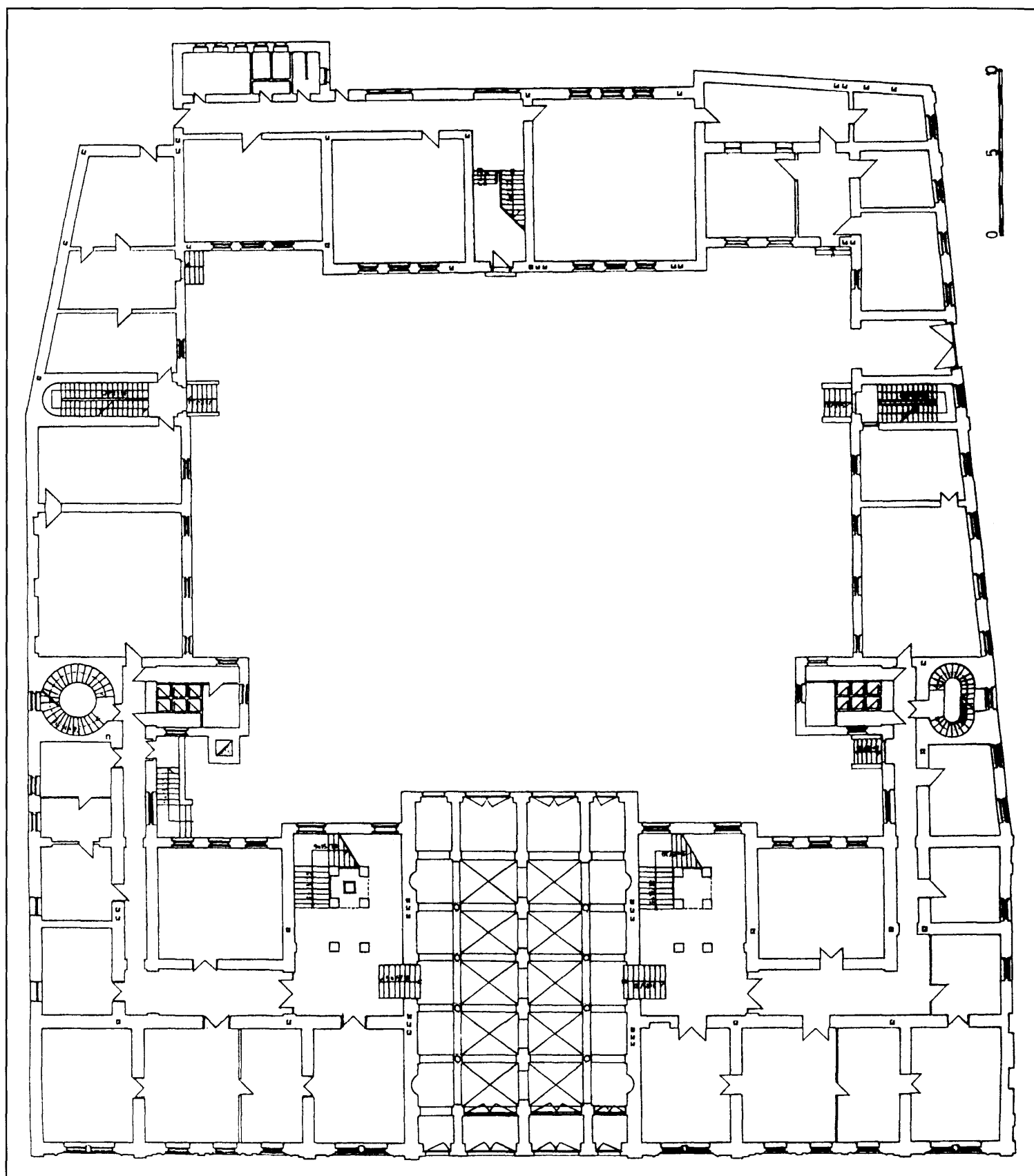
План IV Капетан-Мишино здање (Ректорат Београдског универзитета) – основа приземља
