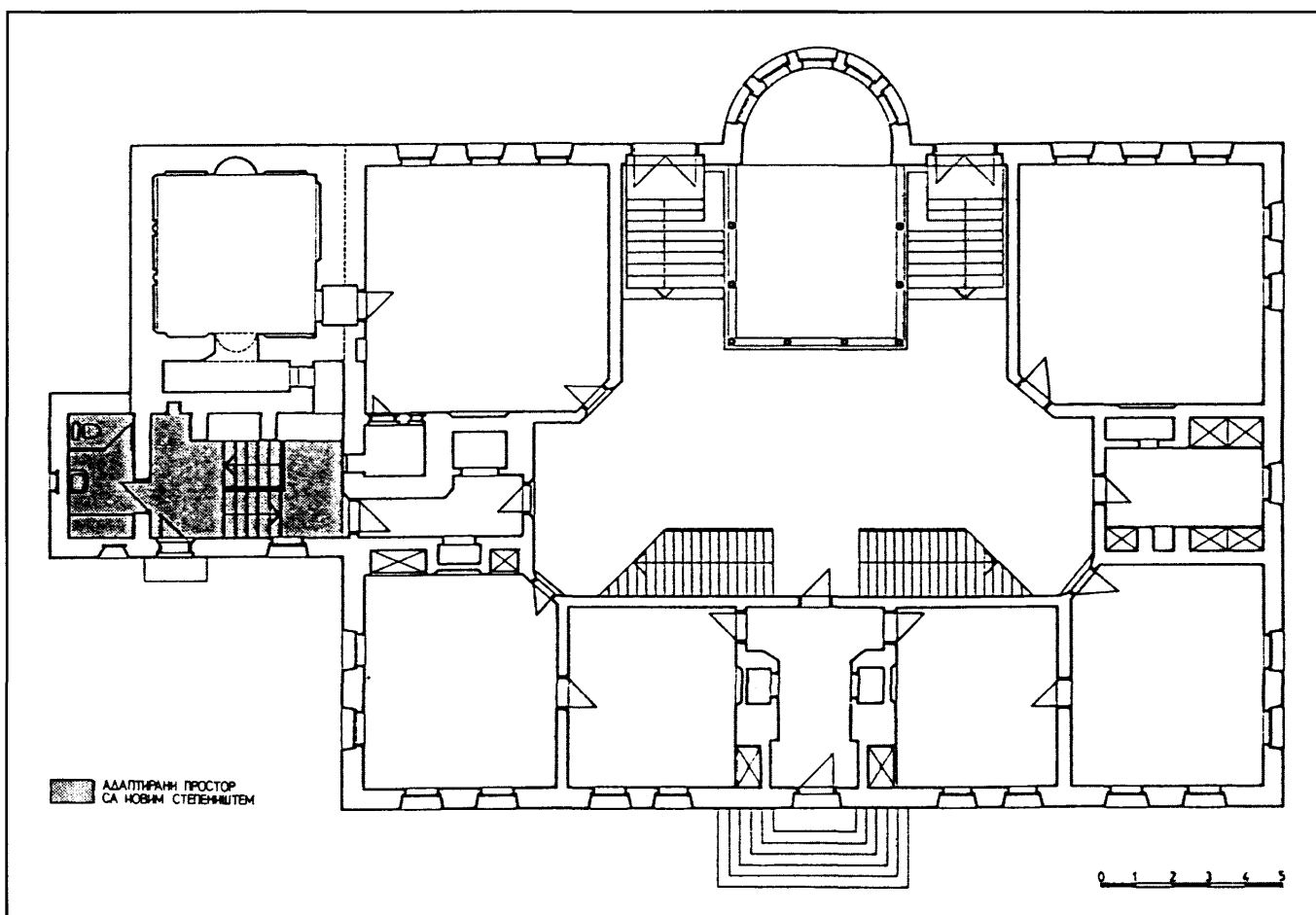
План II
