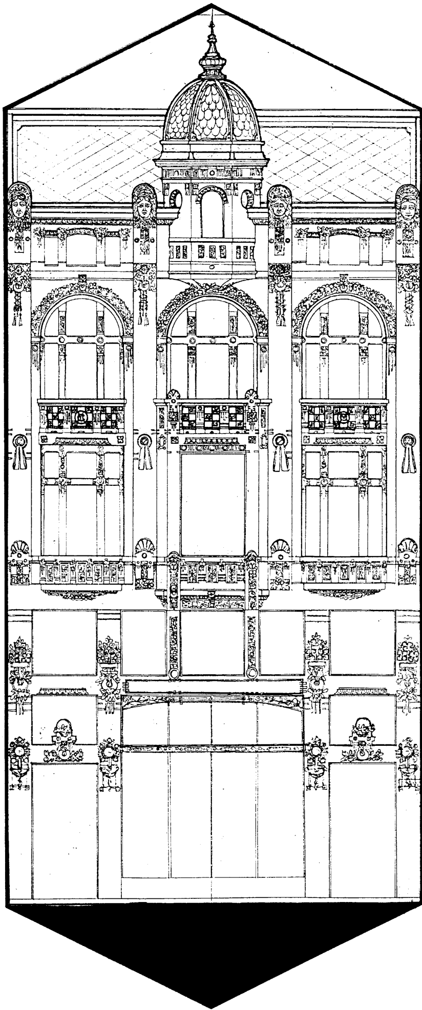
ФАСАДА СМЕДЕРЕВСКЕ КРЕДИТНЕ БАНКЕ, Теразије бр. 39 Подигнута по пројекту арх. Милорада Рувидића 1910. године; Цртеж из пројекта рестаурације фасаде, 1967. год., арх. Зоран Јаковљевић, Док. ЗЗЗСКГБ
