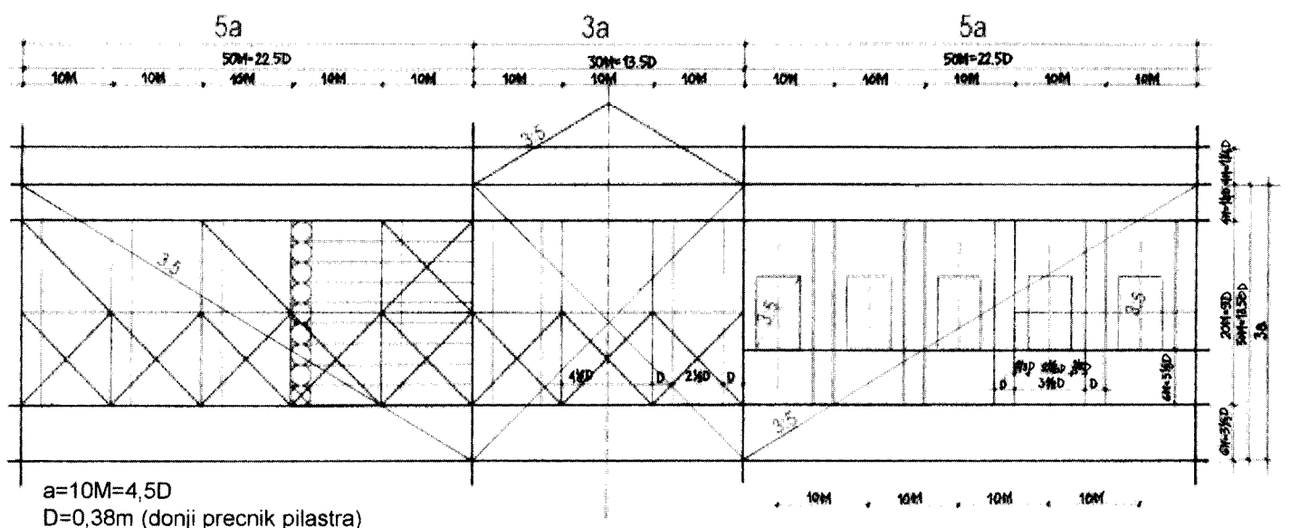
Stilska fasada R 1:100
