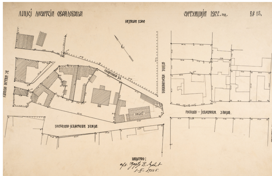
Сл. 9. Ситуација Доситејевој лицеја 1922. године, цртеж арх. Ђорђа Лукића, 1932. (МГБ, Ур_13401)
