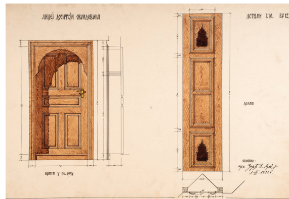
Сл. 8. Враија у њлавном холу и долај Доситејевој лицеја, цртеж арх. Ђорђа Лукића, 1932. (МГБ, Ур_13395)
