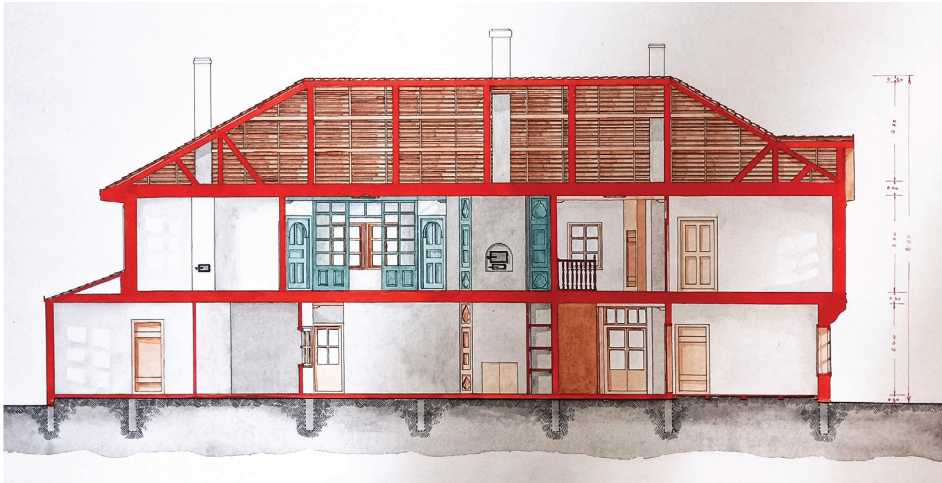
Сл. 4. Пресек Доситејевој лицеја, цртеж Александра Романова, 1931. (МГБ, Ур_4983)
