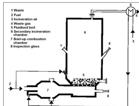
Слика 3. Шема пећи са флуидизованим слојем* * BAT Reference Document for Waste Incineration
