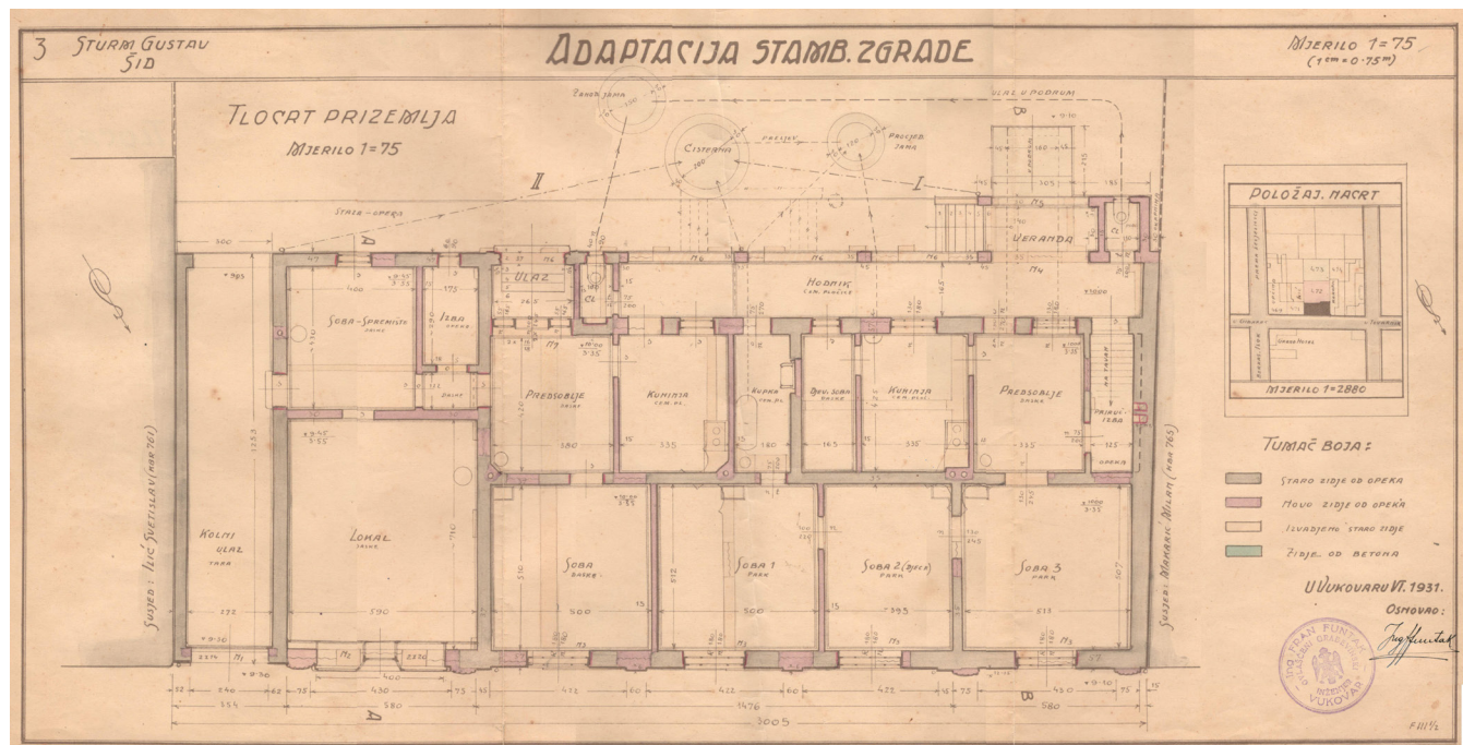
Сл. 3. Основа приземља стамбене зграде Густава Штурма по пројекту Франа Фунтака, 1931. (извор: лична колекција Радована Сремца)
